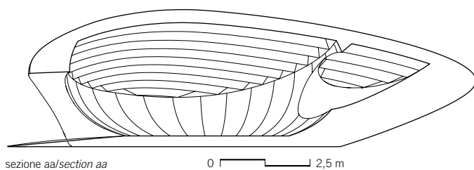
sezione aa/section aa
